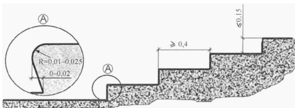
Рисунок 9 - Основные параметры ступеней
