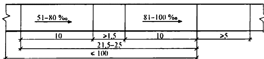
Рисунок 3 - Пример планировки тротуара (пешеходной дорожки)
