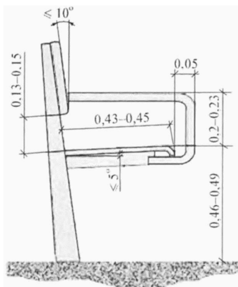
Рисунок Б.5 - Основные параметры уличного кресла (дивана) для инвалидов
