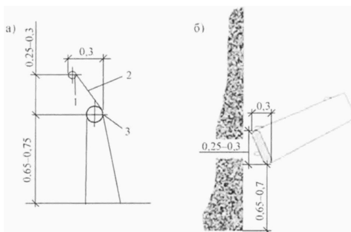
а - поперечный разрез; б - общий вид; 1 - перекладка для поддержки спины; 2 - спинка (сидение); 3 - сиделищная перекладка
