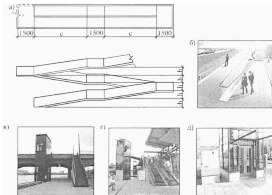
а - типовая схема пандуса; б - размещение пандусов; в, г, д - размещение лифтов; h - высота пандуса; с - длина пандуса
