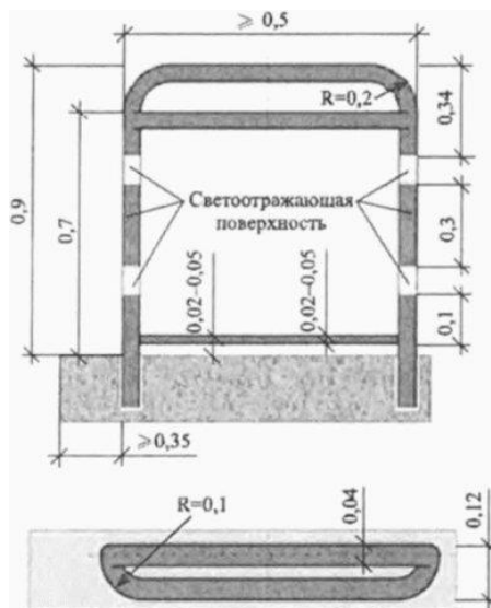
Рисунок 38 - Типовая схема конструкции поручня
