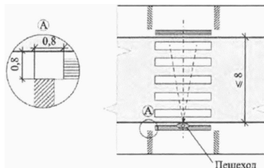
Рисунок 64 - Типовая схема обустройства пешеходного перехода тактильными наземными направляющими указателями
