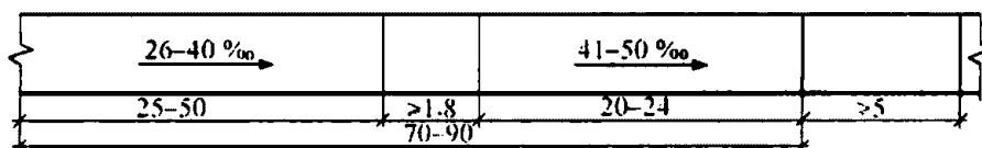
Рисунок 2 - Пример планировки тротуара (пешеходной дорожки) с продольным уклоном, соответствующим нормальным условиям движения инвалидов
