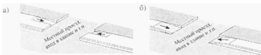
а - пандусы, выполненные по краю тротуара или пешеходной дорожки (комфортные и нормальные условия); б - то же, по ширине тротуара или пешеходной дорожки (стесненные условия)
