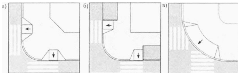
а - пандусы со скошенными боковыми гранями; б - то же, комбинированного типа (в полосе озеленения); в - то же, по ширине переходов
