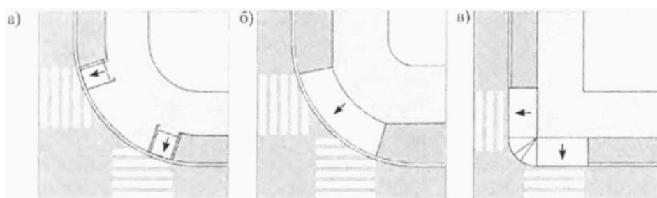
а - пандус на каждом переходе; б - один пандус по ширине внешних границ переходов; в - комбинированный пандус по ширине перехода (уклон \leq 5\text{‰} )
