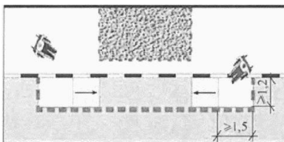
Рисунок 58 - Пример обустройства временного пешеходного пути
