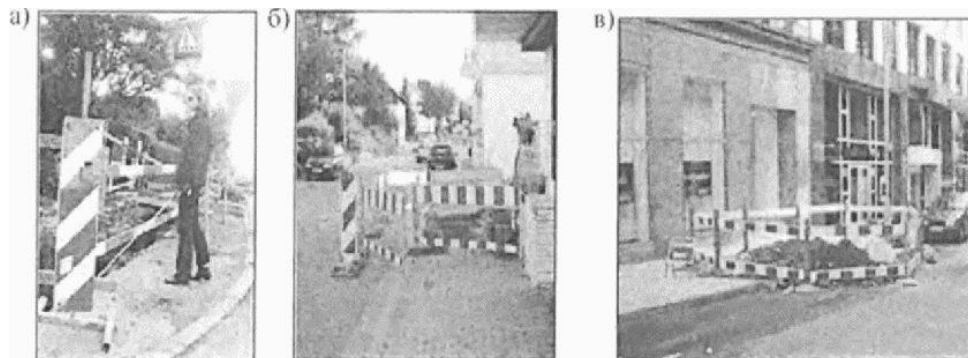
Рисунок 60 - Примеры (а, б, в) обустройства мест проведения дорожных работ ограждениями, обеспечивающими безопасность движения инвалидов
