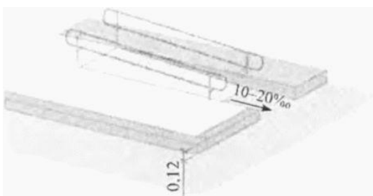
Рисунок 8 - Пример обустройства места резкого перепада высот пешеходного пути на пересечении с проезжей частью дороги
