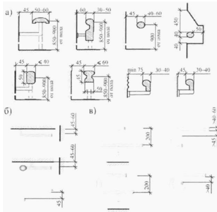
а - параметры поперечного сечения поручней различных типов; б - основные типы элементов, фиксирующих окончание поручней, вид сверху; в - то же, вид сбоку
