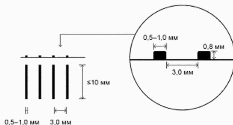
Рисунок 37 — Лестницы
