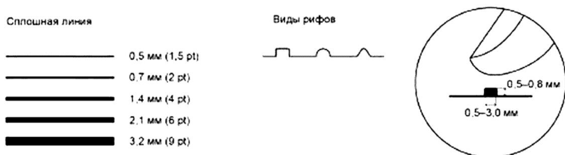
Рисунок 17 — Сплошная линия
