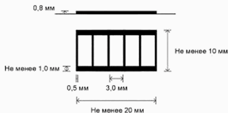
Рисунок 38 — Эскалатор
