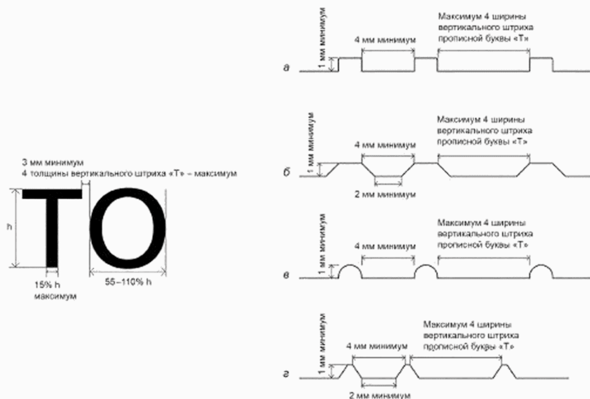
Рисунок 4 — Параметры шрифтовых знаков и рельефа (рифа) РЛШ
