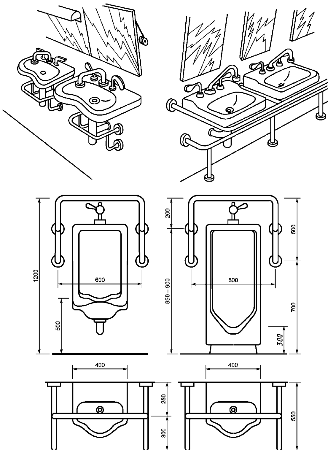
Рисунок 15 - Примеры оборудования поручнями ванных и душевых комнат
