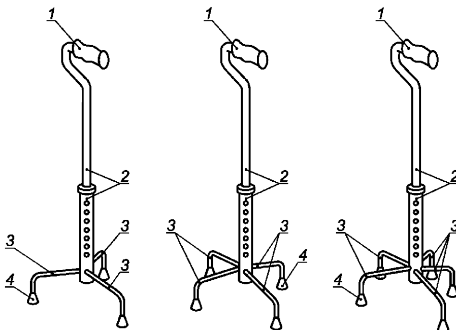
1 - ручка; 2 - стойка; 3 - ножка; 4 - наконечник
