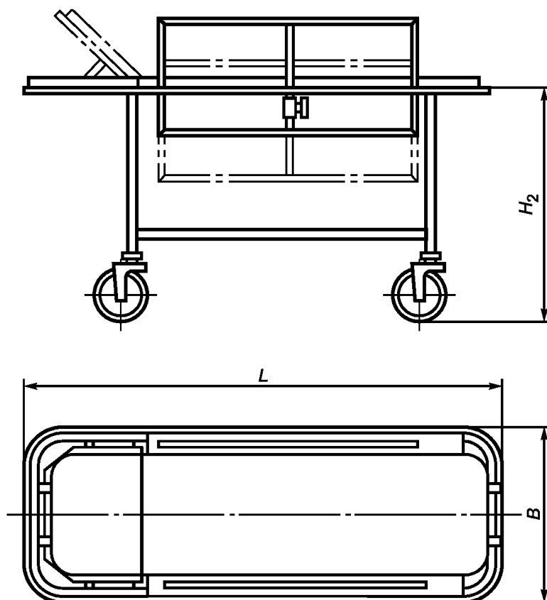
Рисунок 11 - Пример тележки для перевозки детей
