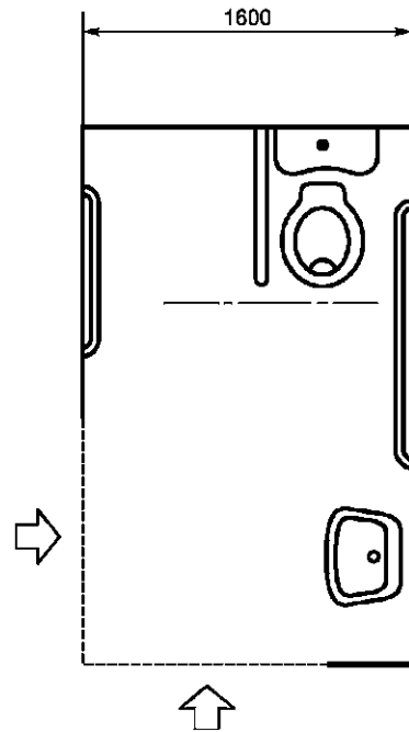
Рисунок 14 - Примеры оборудования поручнями туалетных комнат или кабин
