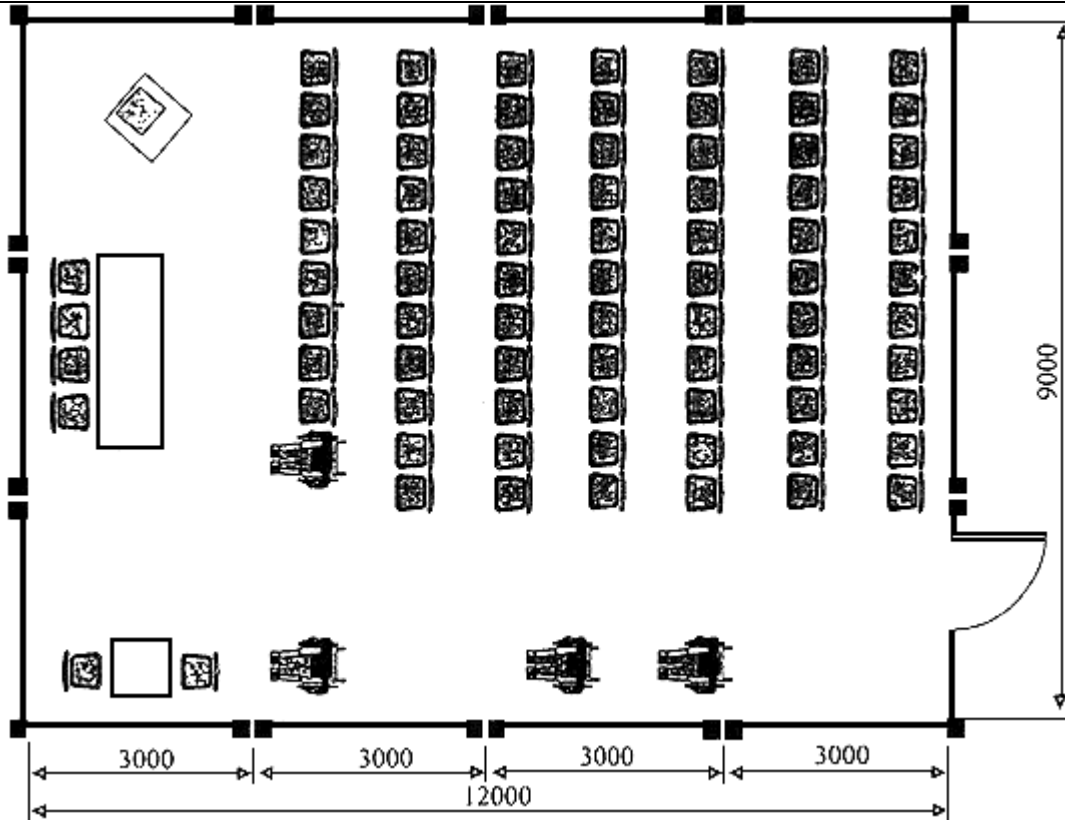
Места инвалидных колясок в помещении для собраний
